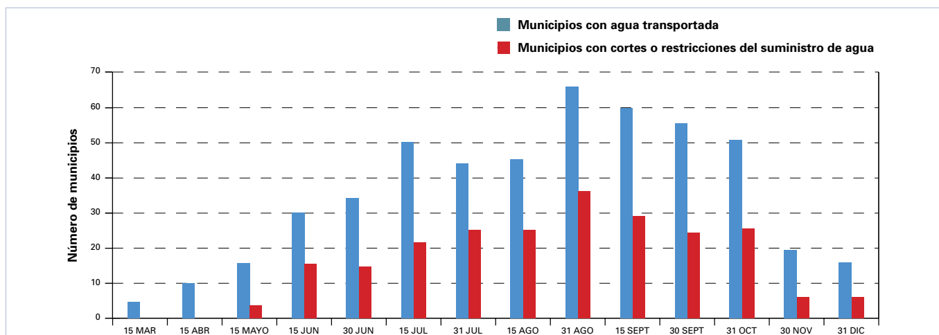
Figura 18. Número de municipios que tuvieron que recurrir a agua transportada (azul) o con restricciones del suministro de agua a los hogares (rojo). (Fuente: Instituto de Meteorología, I.P., Portugal)
