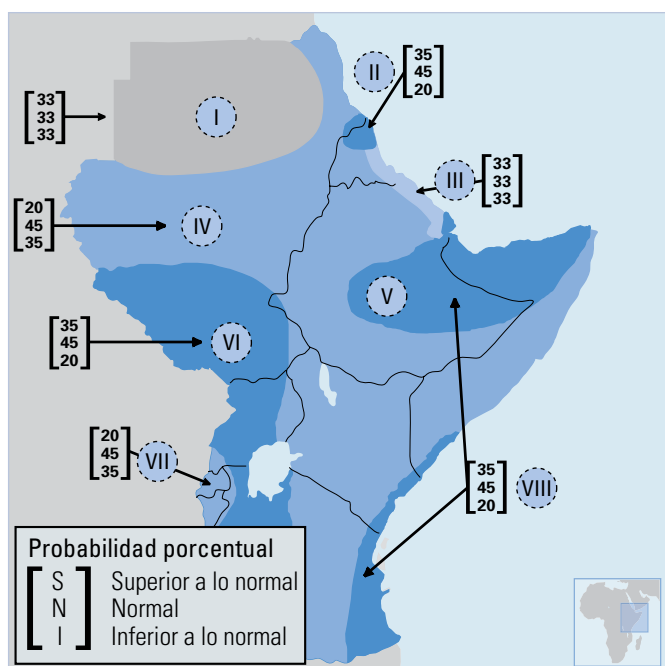
Figura 13. Evolución del clima en la región del Gran Cuerno de África, de marzo a mayo de 2006. (Fuente: ICPAC)
