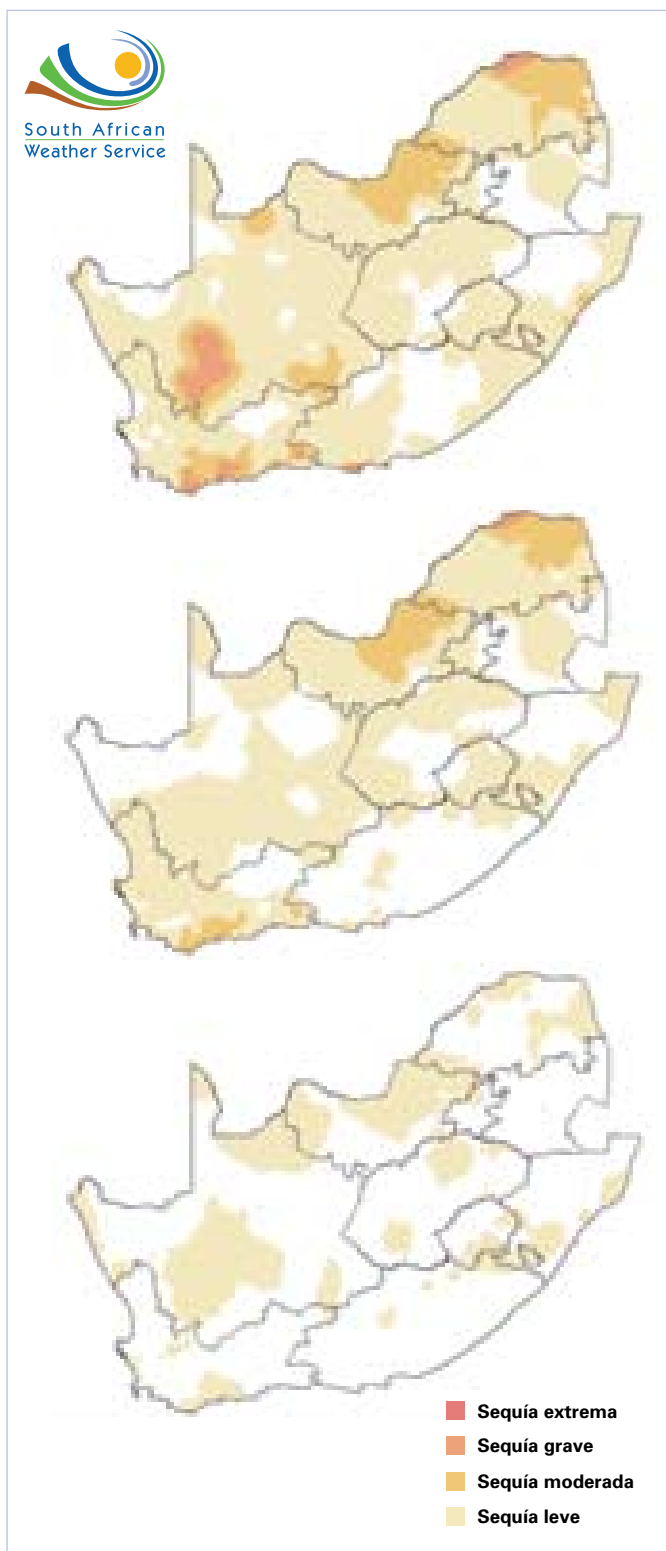
Figura 15. Índice de precipitación normalizado en Sudáfrica, noviembre de 2005 (arriba); de septiembre a noviembre de 2005 (en medio); de junio a noviembre de 2005 (abajo). (Fuente: Servicio Meteorológico de Sudáfrica)
