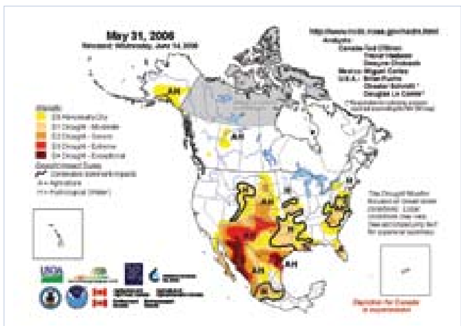
Figura 8. Vigilancia de la sequía de América del Norte, mayo de 2006 (Fuente: Vigilancia de la sequía de América del Norte, http://www.ncdc.noaa.gov/oa/climate/monitoring/drought/nadm/index.html )
