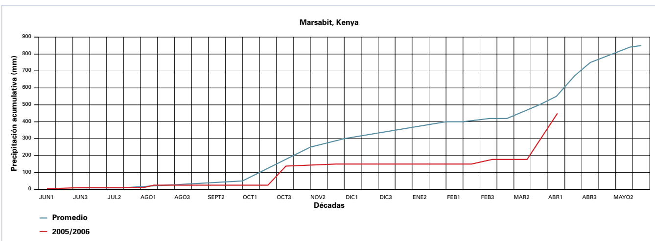
Figura 12. Ejemplos de precipitación de lluvia decadal acumulativa en partes de Kenya entre junio de 2005 y principios de abril de 2006. (Fuente: ICPAC)
