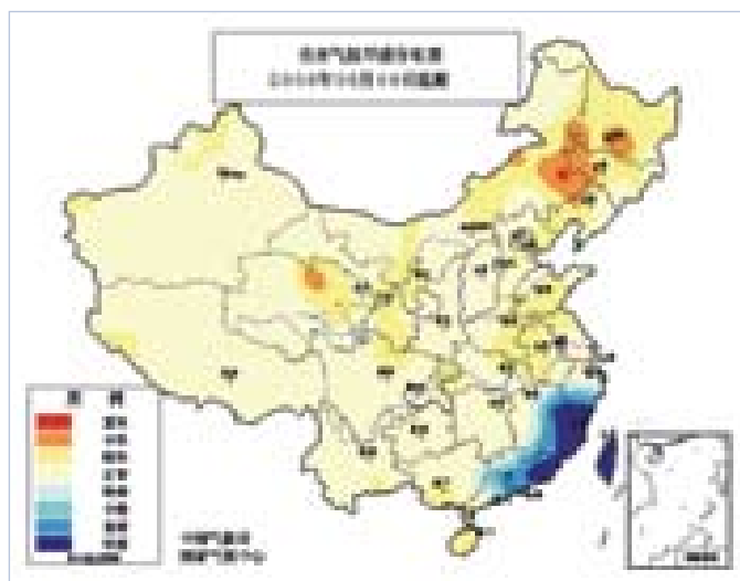
Figura 9. Vigilancia de la sequía en China, 9 de junio de 2006; la escala de colores de beige (en el centro) a rojo denota niveles de gravedad crecientes de sequía. (Fuente: Administración Meteorológica China)
