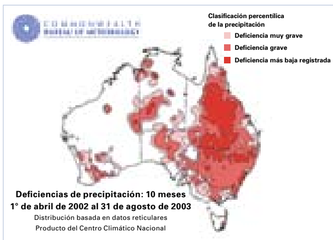
Figura 19. Extensión de las deficiencias de precipitación graves o más graves en el momento de mayor intensidad del último episodio de sequía relacionado con El Niño, en 2002 y 2003. (Fuente: Oficina de Meteorología de Australia)
